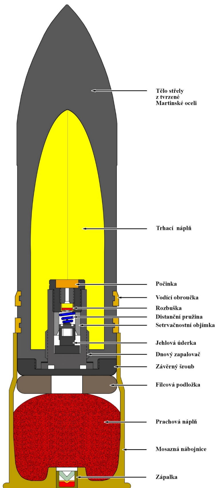
37 mm Granatpatronen M. 15
